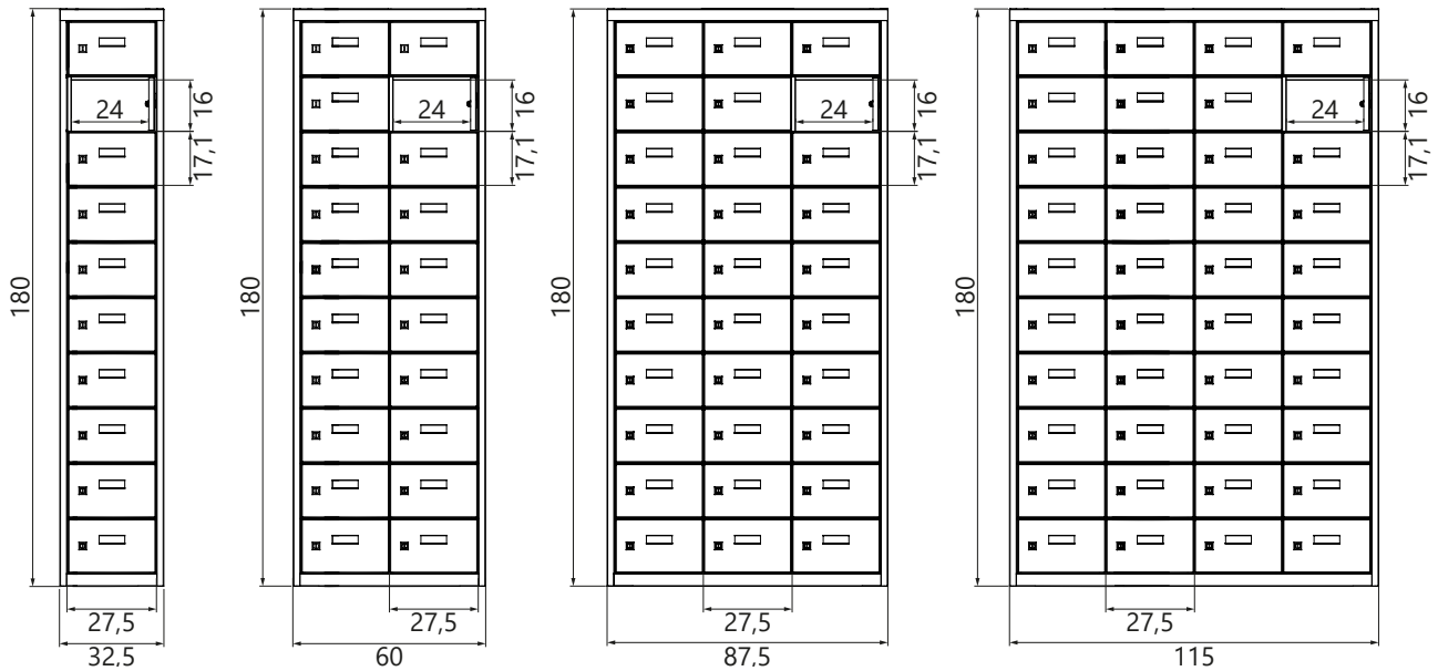
Fachbreite 27,5 cm
